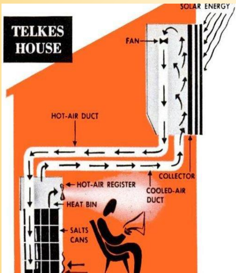
Esquema del funcionamiento de la casa Telkes.
